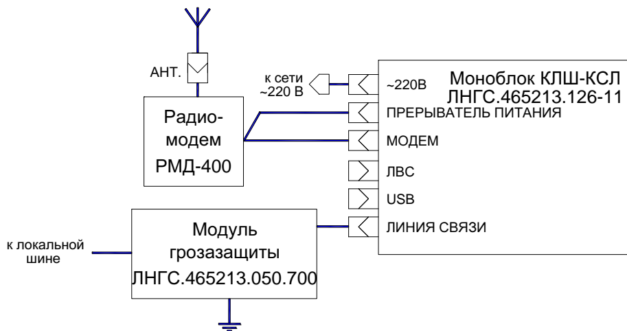
Рисунок 2. Схема подключения моноблока КЛШ-КСЛ СМ3 433 МГц (ЛНГС.465213.126-11)
