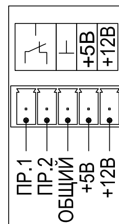
Рисунок 2. Назначение контактов разъема «Прерыватель питания»
