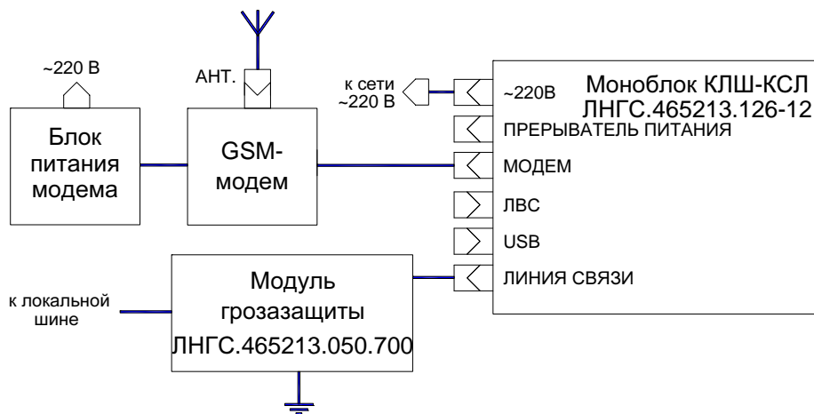
Рисунок 3. Схема подключения моноблока КЛШ-КСЛ СМ3 GSM (ЛНГС.465213.126-12)
