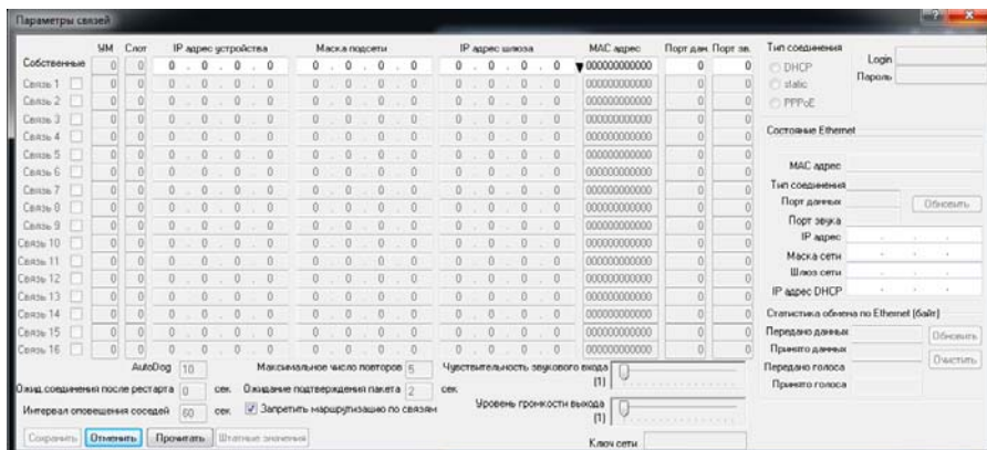
Рисунок 5. Диалоговое окно параметров связей КСЛ моноблока
