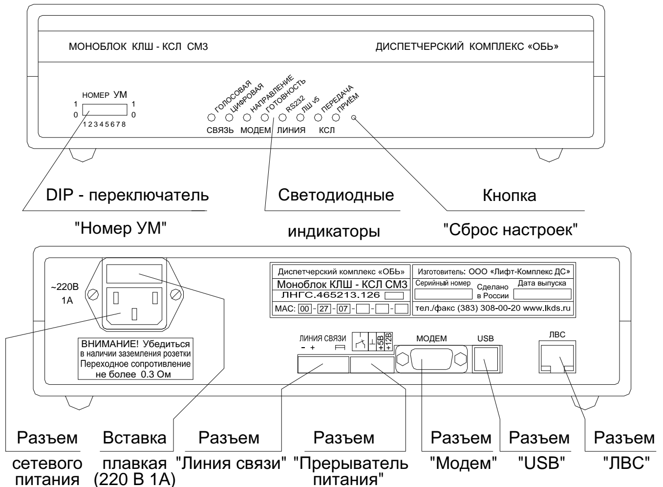
Рисунок 1. Внешний вид моноблока КЛШ-КСЛ СМЗ
