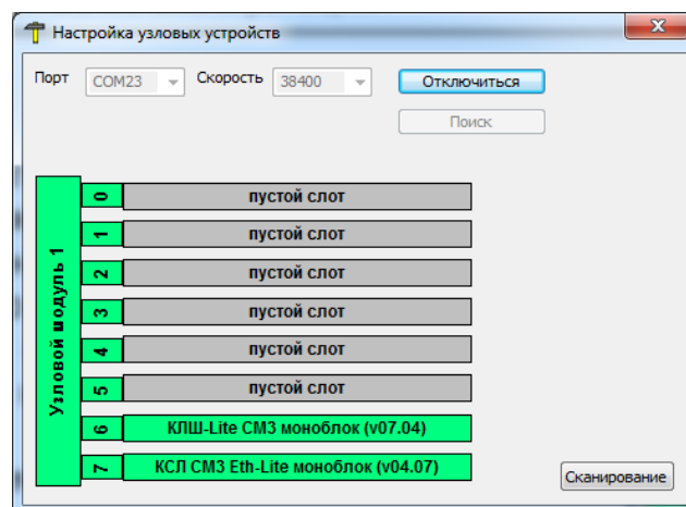
Рисунок 4. Диалоговое окно программы после подключения к моноблоку
