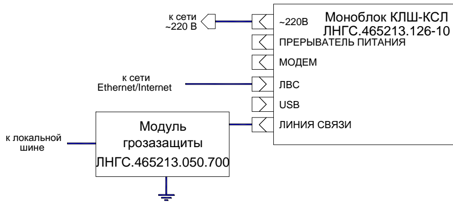
Рисунок 1. Схема подключения моноблока КЛШ-КСЛ СМ3 Ethernet (ЛНГС.465213.126-10)
